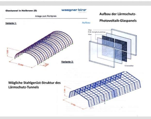
Halbrunder (elliptischer) Querschnitt oder aus ebenen Flächen
